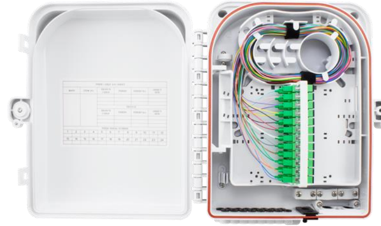
24 port
